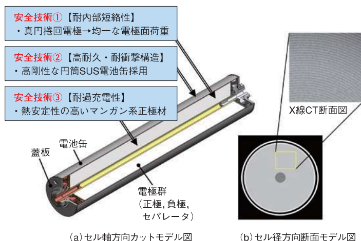
図7 リチウムイオン電池CH75セルの安全技術
