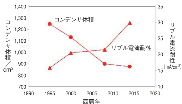
図10 当社ネジ端子形アルミ電解コンデンサの製品体積とリップル電流耐性の推移(定格450 V, 6800 \mu\text{F} )
